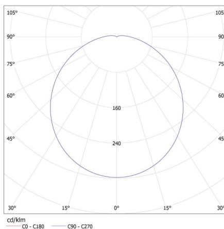
MILED0 (kat 30412) DUNO LED 24W-WW-O / Krzywa rozsyłu światła (biegunowo)
