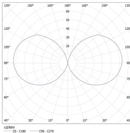
KANLUX S.A. (kat 25680) SORTA 30I-UP / Krzywa rozsyłu światła (biegunowo)
