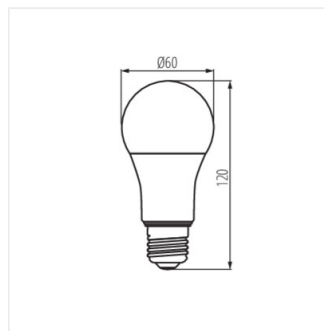
IQ-LEDDIM A6012,5W, IQ-LEDDIM A60 15W
