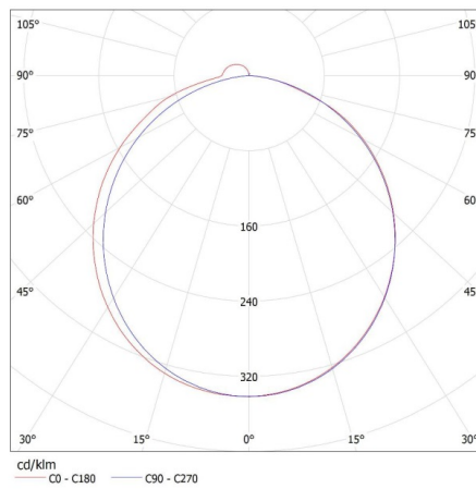
KANLUX S.A. (kat 26681) ASTEN LED IP44-12W-NW / Krzywa rozsyłu światła (biegunowo)
