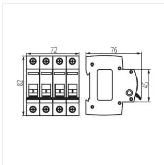
KMI-4/63A
