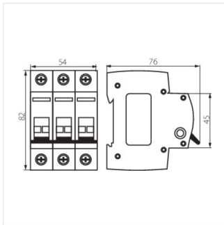
KMI-3/80A
