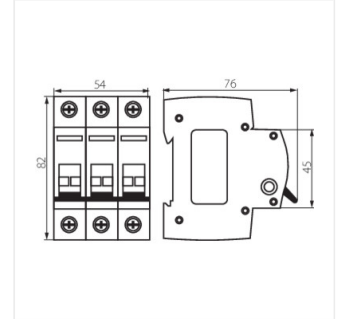
KMI-3/63A
