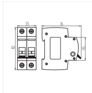
KMI-2/40A
