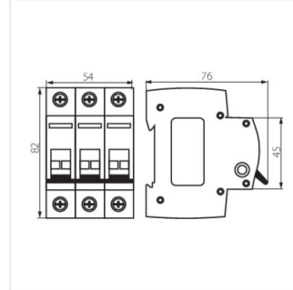
KMI-3/40A
