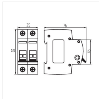
KMI-2/25A
