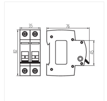
KMI-2/63A
