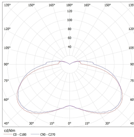
KANLUX S.A. (kat 27378) APUS LED W-NW / LDC (Polar)
