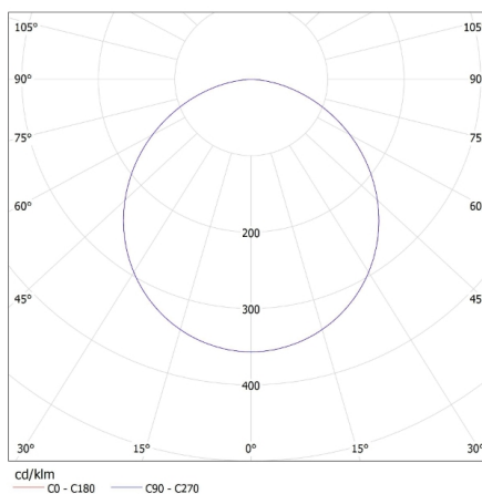
MILEDO (kat 31083) SP LED N 18W NW-R / LDC (Polar)
